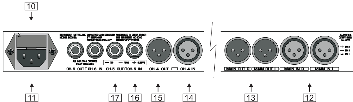
Fig. 3.3 : Éléments du panneau arrière de l'ULTRALINK PRO MX882
